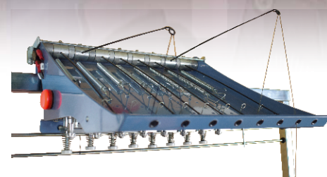
Tensionatore a 8 antenne Tightener with 8 antennas
